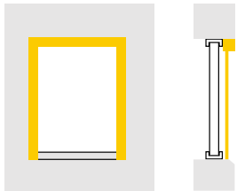
Winsol : SolarFix & SolFix 90 RE intégrés dans le jour
