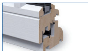
Carrelet lamellé-collé abouté 3 plis en essence haute densité
