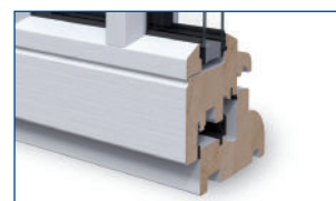
Ouvrant et dormant de 68 mm d'épaisseur
